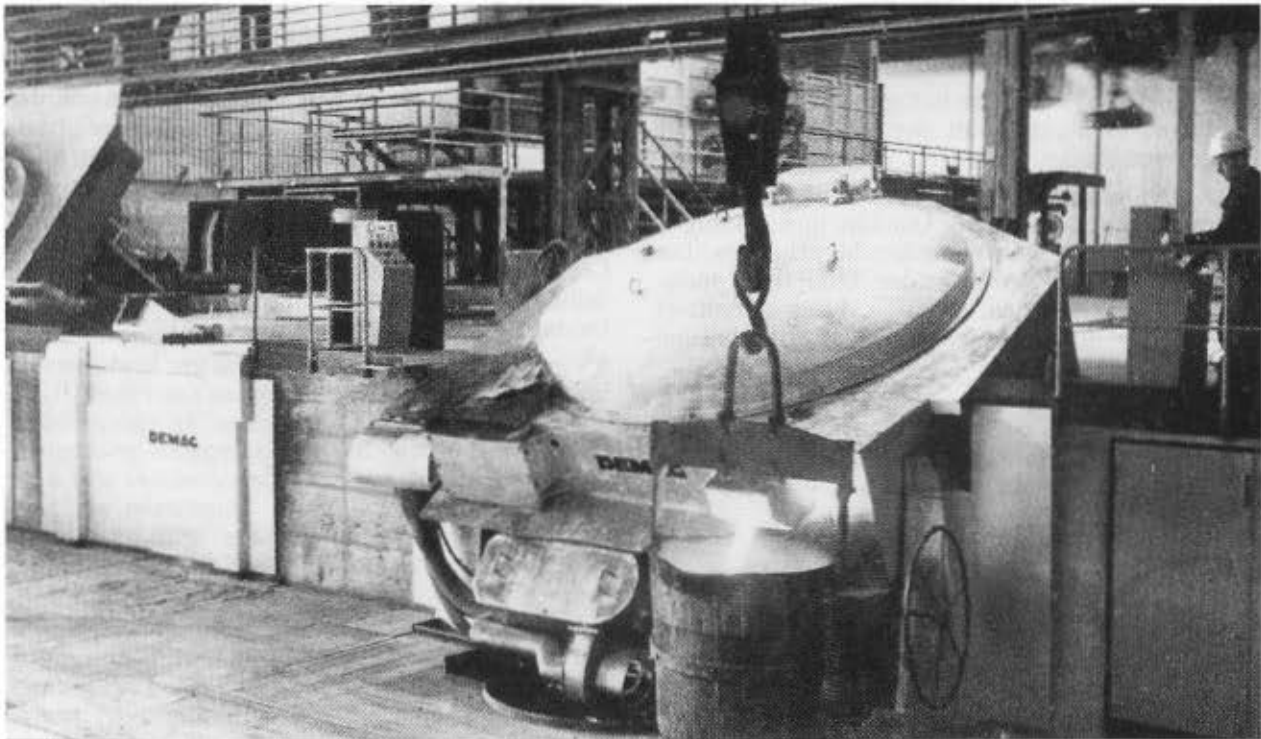
Der Elektroschmelzofenbetrieb mit Induktionstiegelofen (links); die Gießpfanne wird aus dem als Warmhalteofen verwendeten Induktionsrinnenofen gefüllt /31/.
