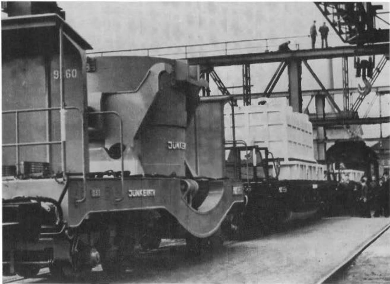
Ein Zug aus Hüttenfahrzeugen im Werksgelände. Im Vordergrund Roheisenpfannenwagen. Solche Fahrzeuge gingen von Jünkerath aus in die ganze Welt /33/.
